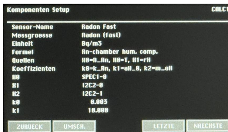
Abbildung 7: Komponenten-Konfiguration
