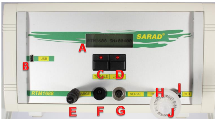
Abbildung 1: Anschlüsse und Bedienelemente
